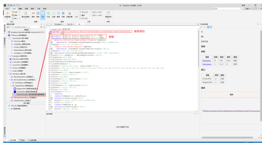
图 4-5 阻感负载模型代码编写
