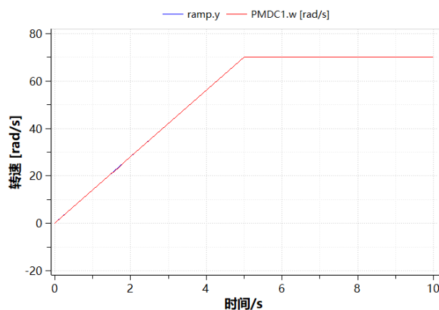
图 5-4 转速跟踪曲线
