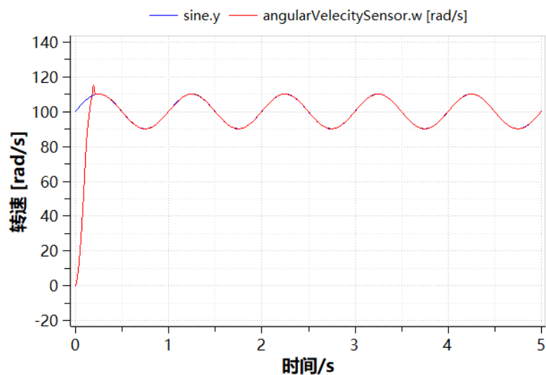
图 5-8 转速跟踪曲线
