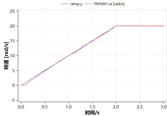
图 5-6 转速跟踪曲线
