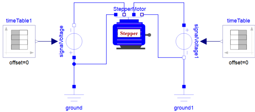
图 5-9 步进电机系统
