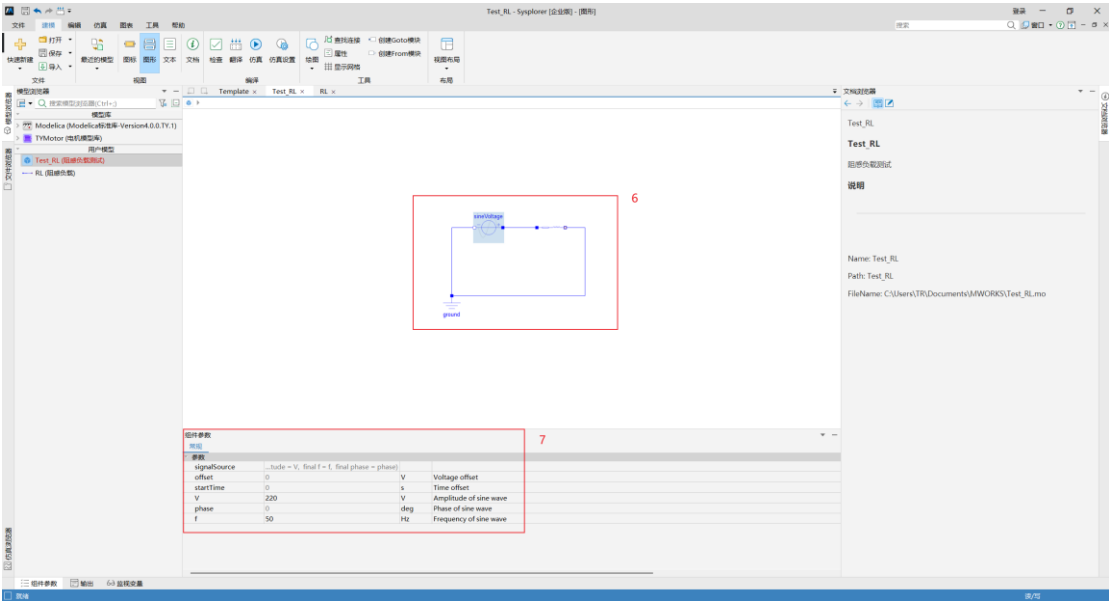
图 4-10 接口连线搭建系统模型以及参数设置
