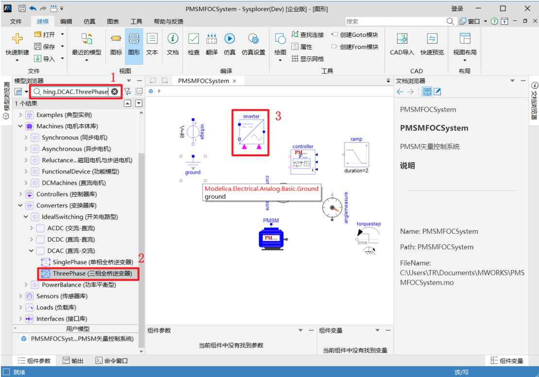
图 3-4 新建模型（方式一）
