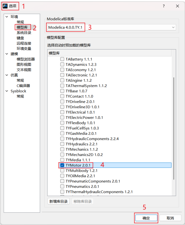
图 2-14 模型库加载（方式二）
