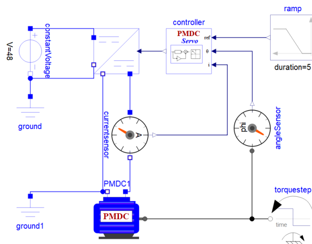
图 5-3 永磁直流电机系统
