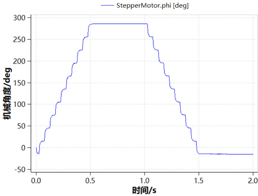
图 5-10 机械角度曲线
