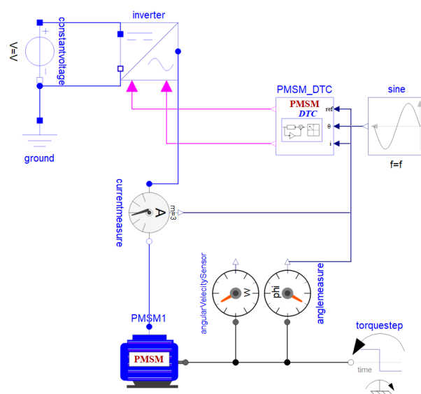
图 5-7 永磁同步电机 DTC 系统
