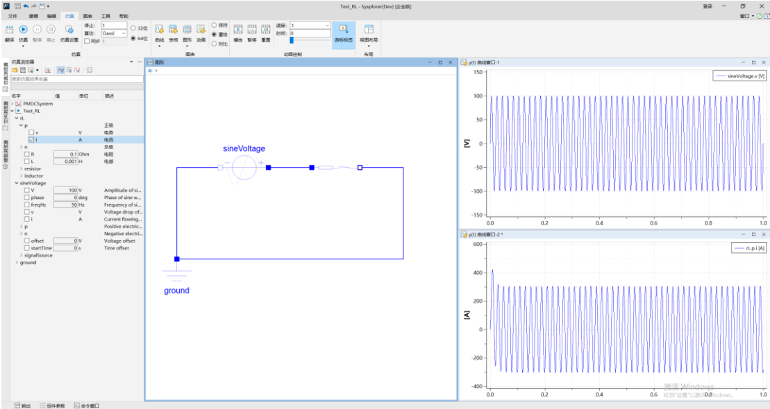
图 4-15 阻感负载测试系统仿真结果展示
