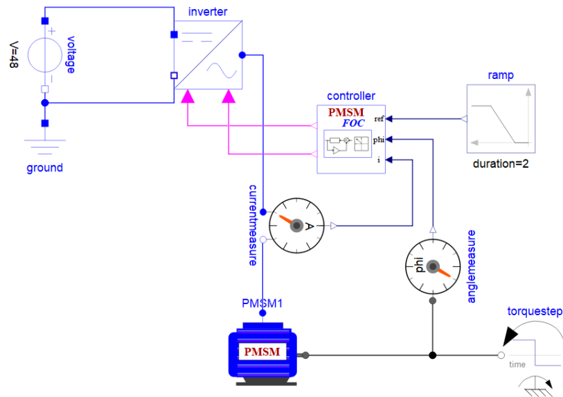
图 5-5 永磁同步电机 FOC 系统
