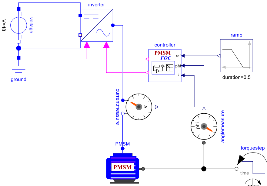
图 3-2 PMSM 速度控制系统模型
