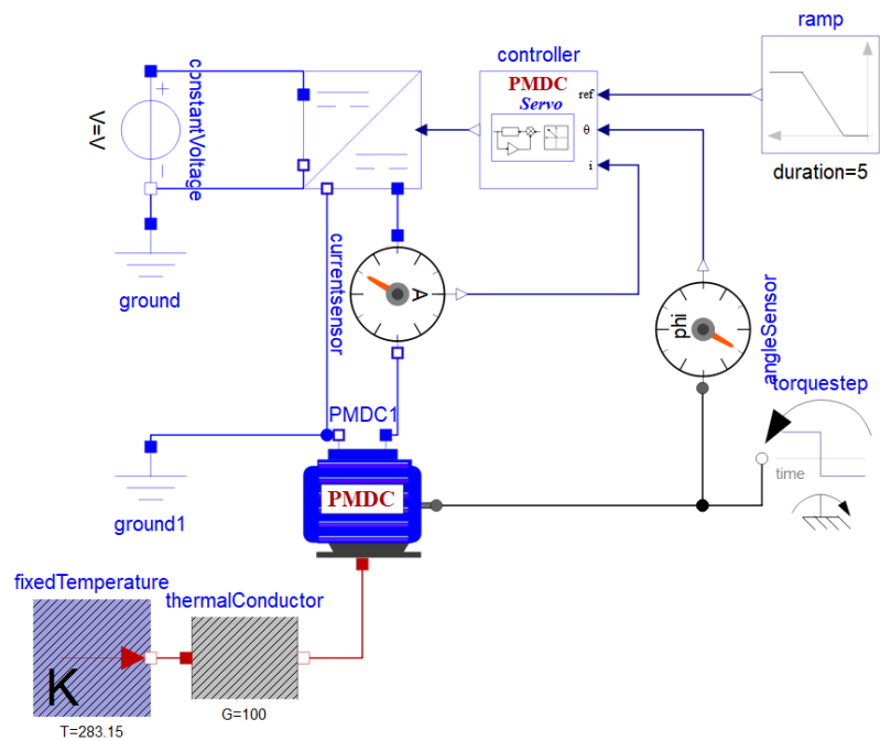
图 5-11 电机冷却系统
