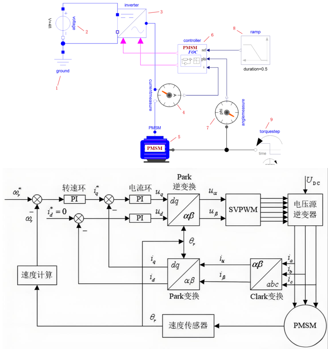
图 3-1 PMSM 矢量控制系统基本架构
