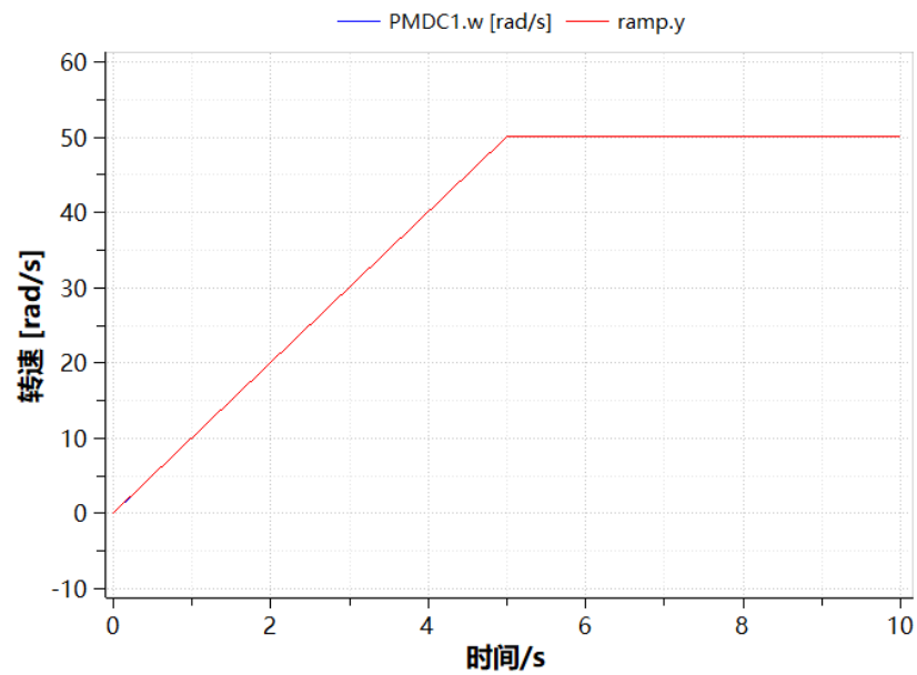
图 5-12 转速跟踪曲线
