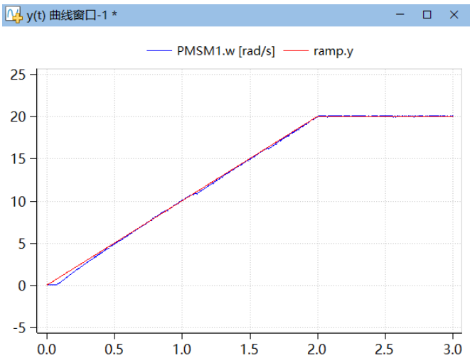
图 3-8 PMSM 控制系统速度跟随曲线
