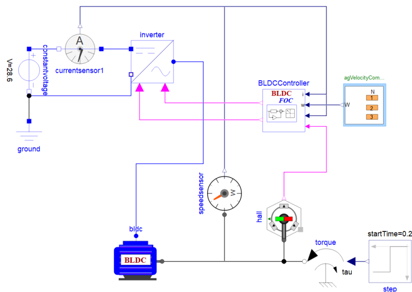
图 5-1 无刷直流电机系统
